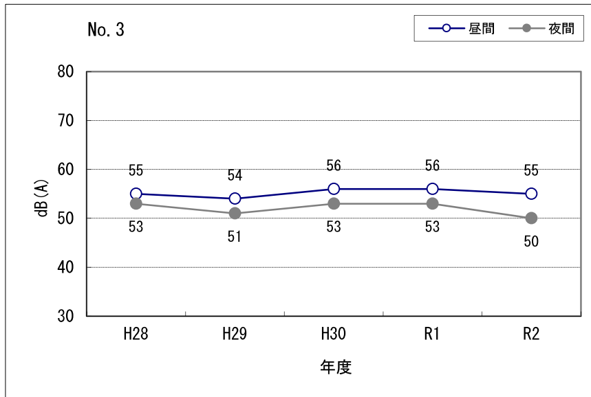
図 II-5.1 等価騒音レベルの経年変化 (No. 3)
