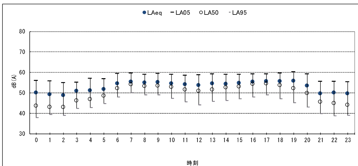
図Ⅱ-3.1 騒音レベル経時変化
