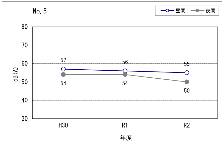
図 II-5.3 等価騒音レベルの経年変化 (No. 5)
