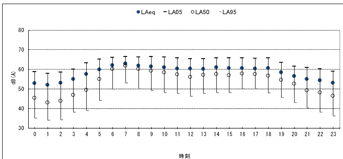
図Ⅱ-3.4 騒音レベル経時変化
