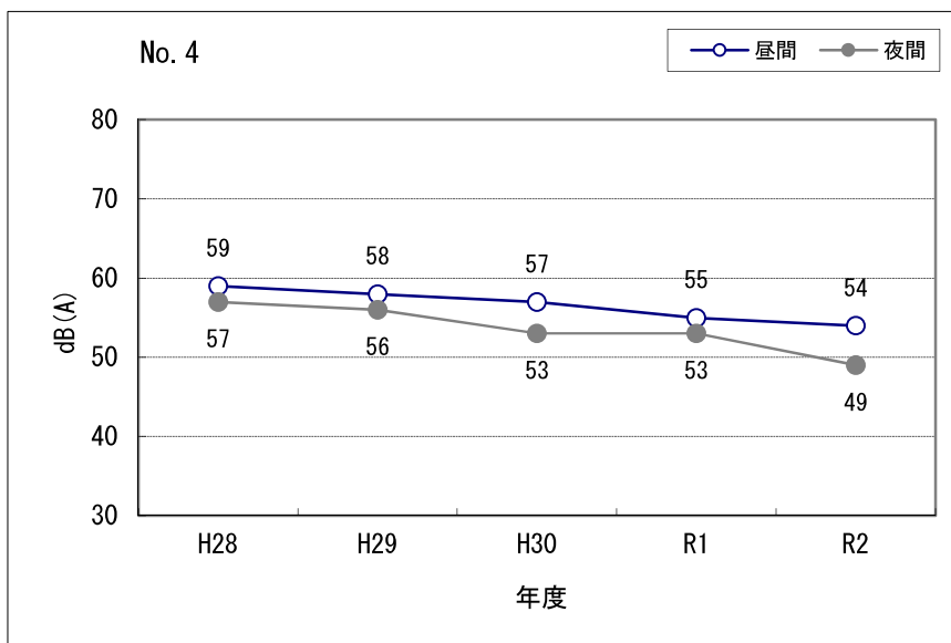
図 II-5.2 等価騒音レベルの経年変化 (No. 4)
