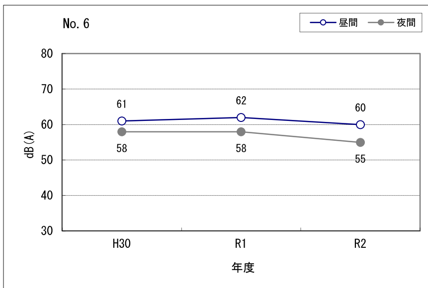
図 II-5.4 等価騒音レベルの経年変化 (No. 6)
