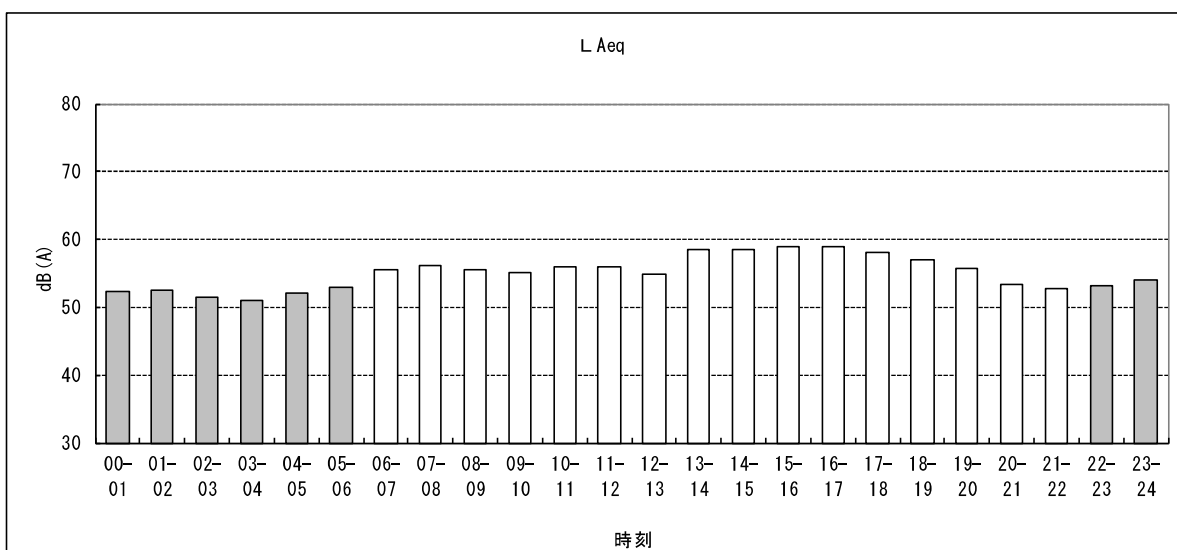
図Ⅱ-3.2 等価騒音レベル経時変化
