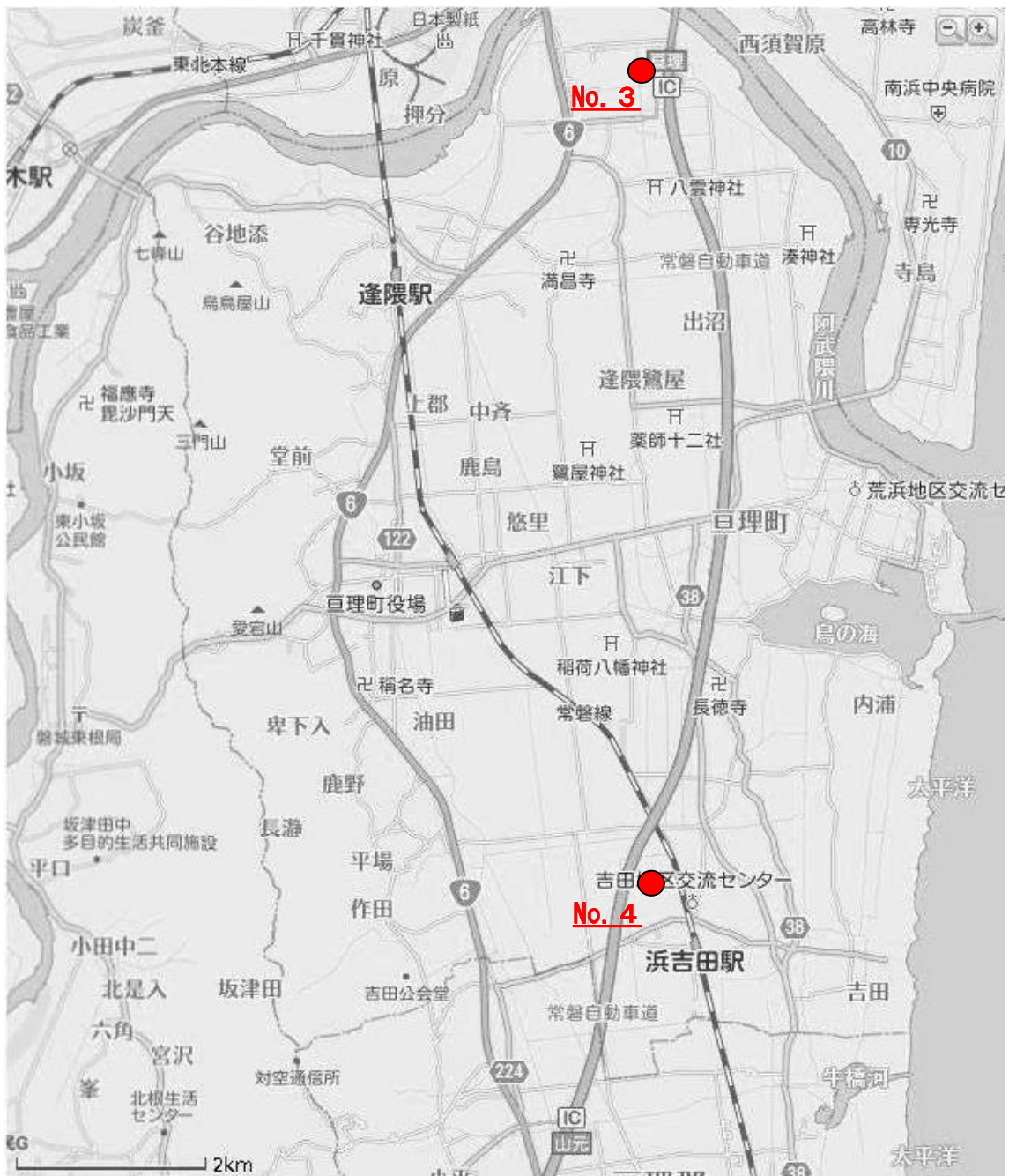
図 II -1 自動車交通騒音調査地点位置図
